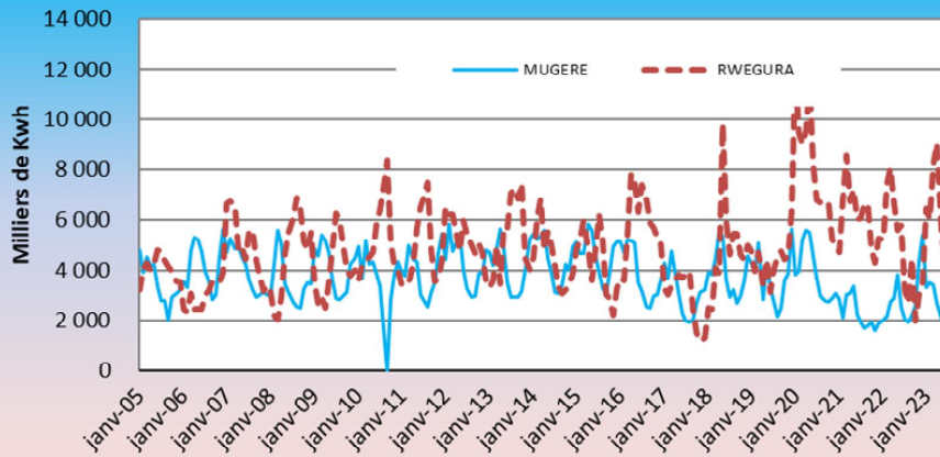
Evolution mensuelle de la production d'électricité à MUGERE et RWEGURA
