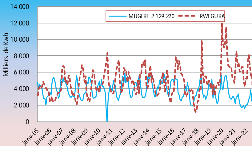
Evolution mensuelle de la production d'électricité à MUGERE et RWEGURA
