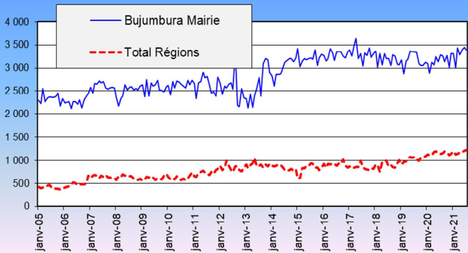
Evolution de la production d'eau, à Bujumbura et dans les régions en milliers de m 3
