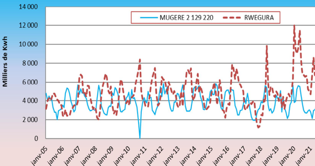
Evolution mensuelle de la production d'électricité à MUGERE et RWEGURA
