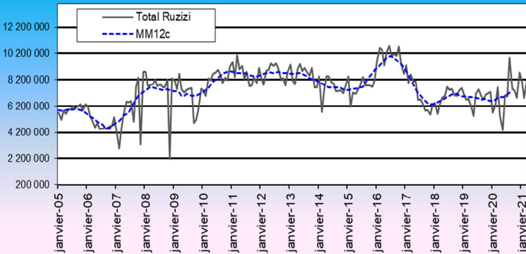
Evolution d'électricité en provenance de RUZIZI I et II en kw/h
