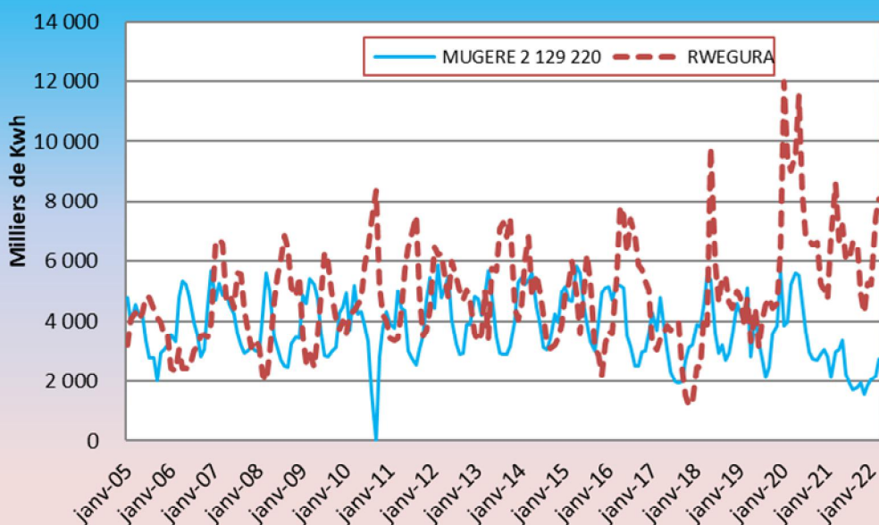
Evolution mensuelle de la production d'électricité à MUGERE et RWEGURA
