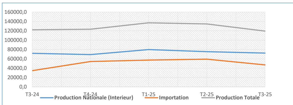
Graphique 3. Evolution de la production et importation trimestrielles de l'énergie électrique (milliers KWh)
