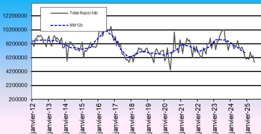
Evolution d'électricité en provenance de RUZIZI I et II en kw/h
