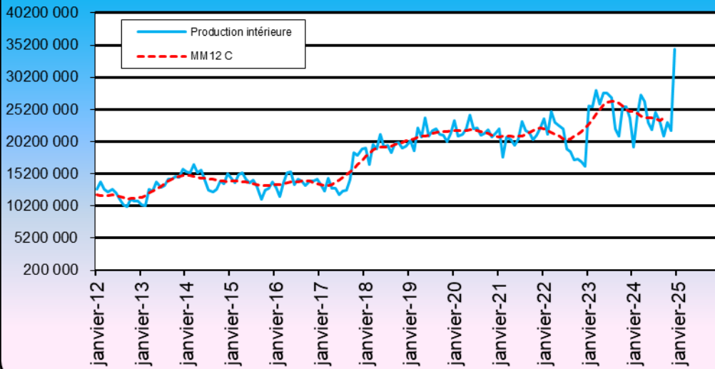
Evolution de la production intérieure d'électricité en kw/h
